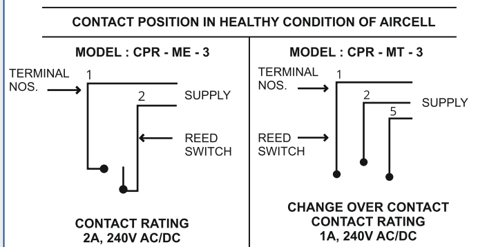
FIG 3. WIRING DIAGRAM
